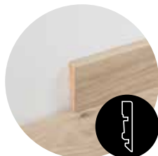
Plinthes assorties de 60 mm Installation : colle ou clips 2400 x 12 x 60 mm (L x l x H)
